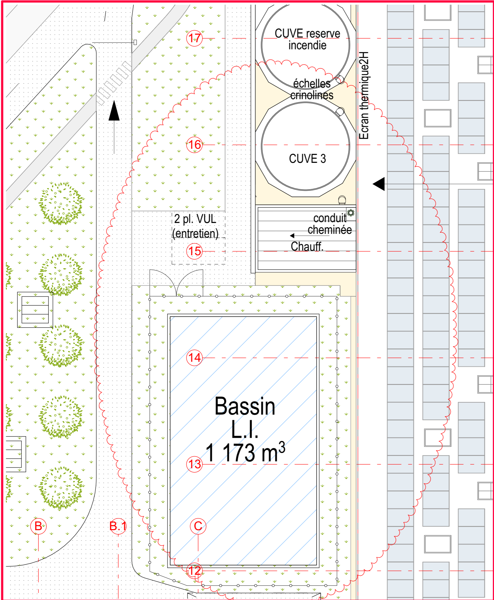
agrandissement sur la cuve 3 1:250°
